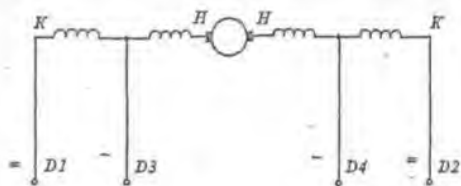
Рис. 1 Электрическая схема соединения обмоток электродвигателя ДКУ для правого направления вращения.
