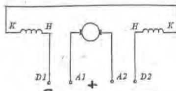
Рис. 2 Электрическая схема соединения обмоток электродвигателя ДП для реверсивного направления вращения.
