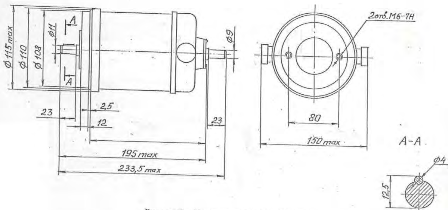
Рисунок 3 - Исполнения ИМ3601 – ИМ3602
