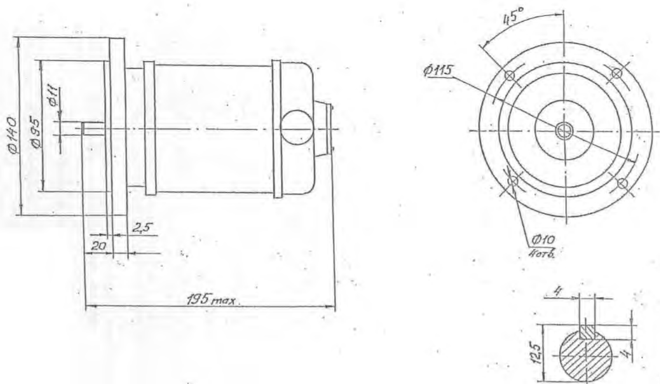
Рисунок 5 - Исполнение IM3001
